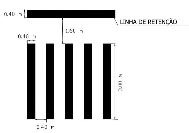
Detalhamento faixa travessia de pedestres *sem escala
