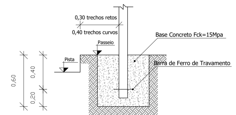
Detalhamento fixação das placas *sem escala
