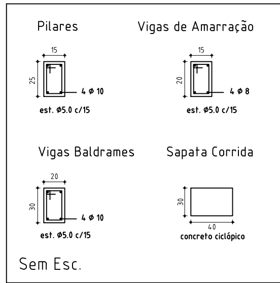
CORTE ESQUEMÁTICO:
