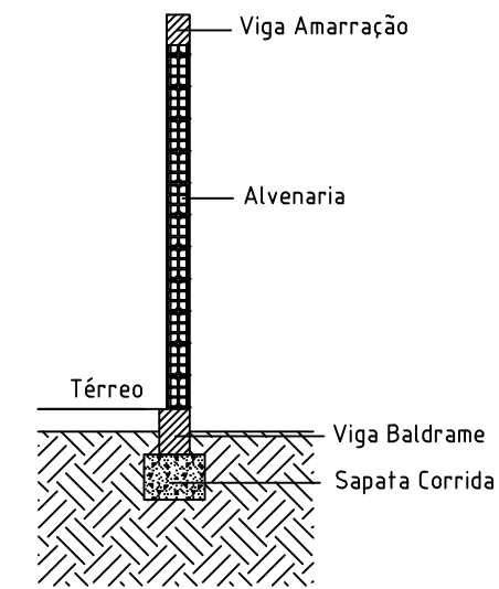
CORTE ESQUEMÁTICO:
