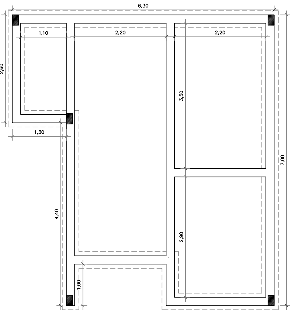
PROJETO ESTRUTURAL
