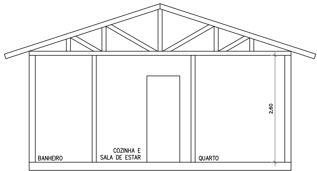
CORTE AA'
