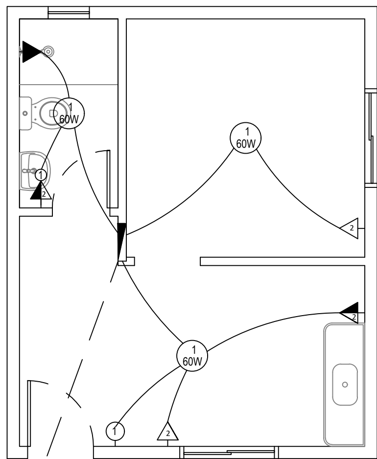
PROJETO ELÉTRICO
