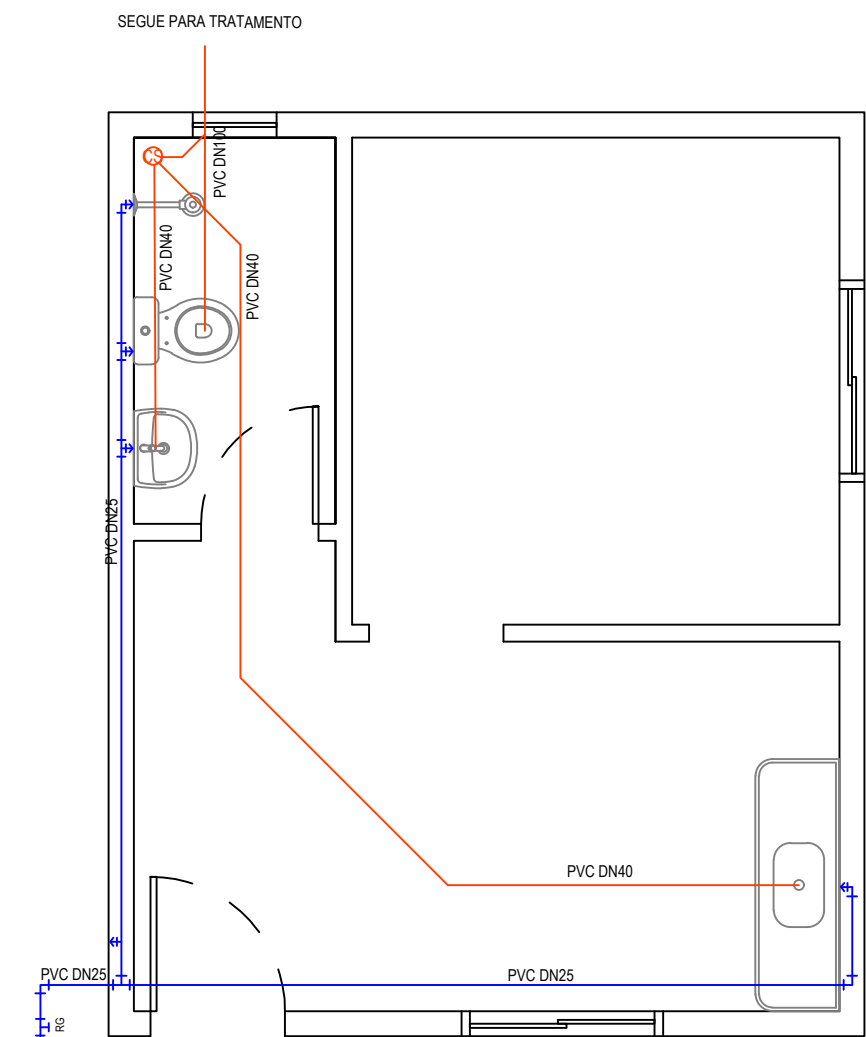
PROJETO HIDROSSANITÁRIO
