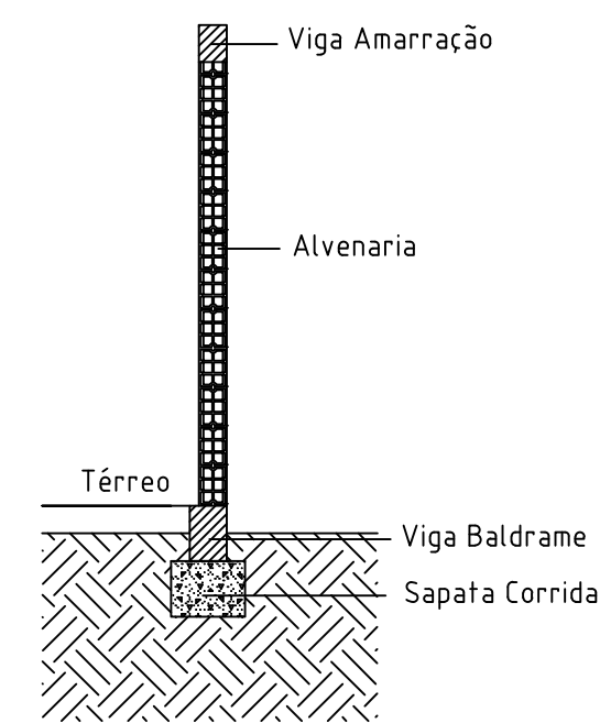
CORTE ESQUEMÁTICO:
