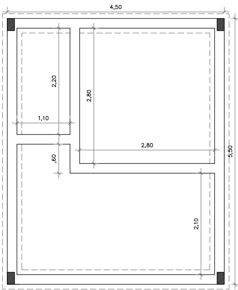
Sapatas, Vigas Baldrame e Pilares
