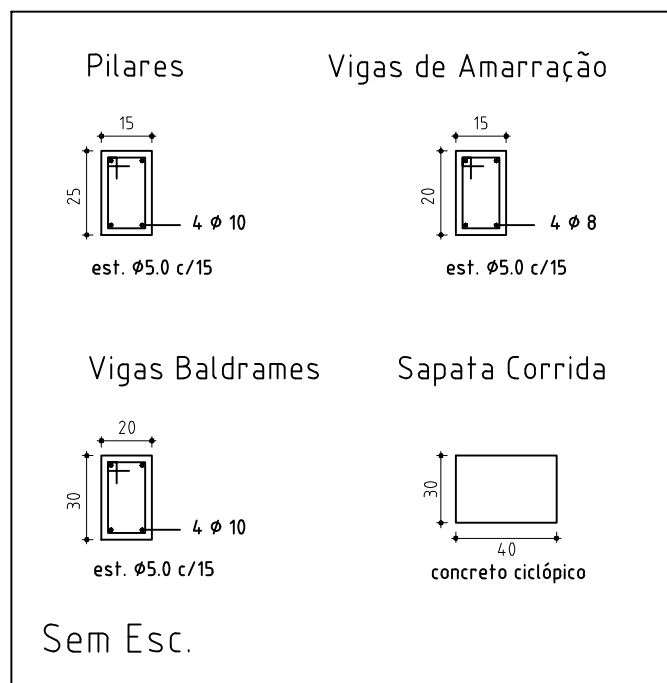
CORTE ESQUEMÁTICO:
