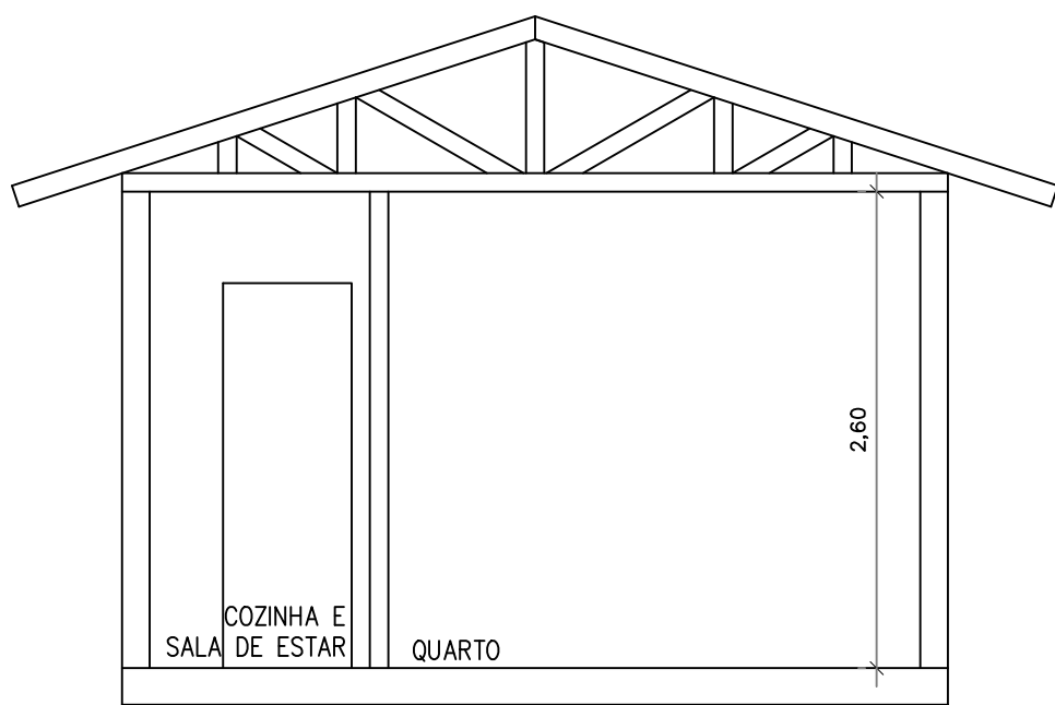
CORTE AA'
