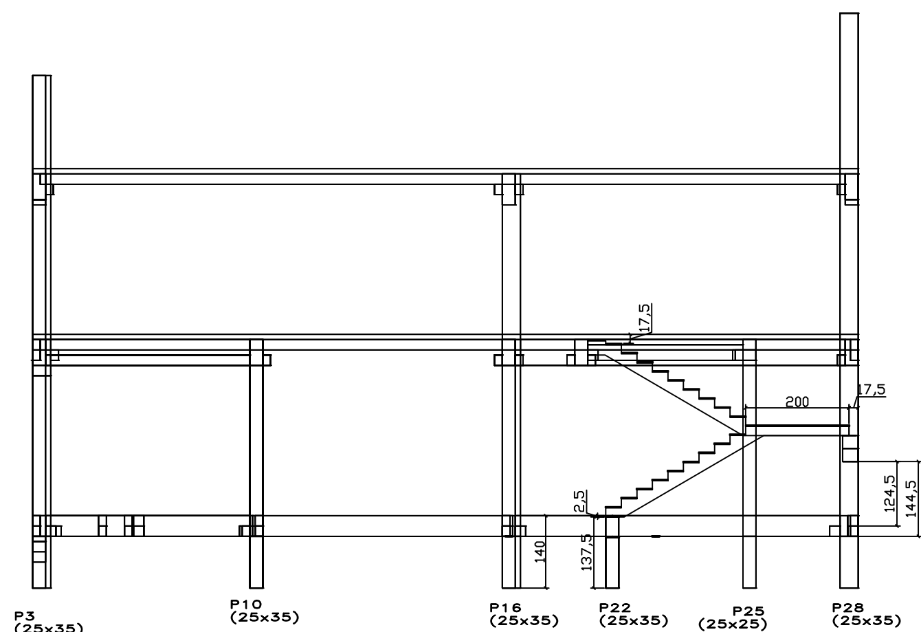
Corte Detalhe Escada
