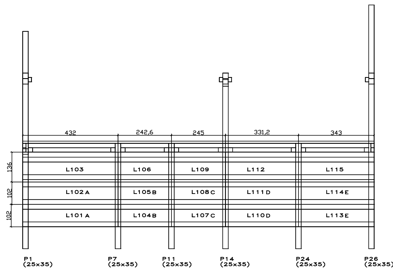
Corte Numeração Lajes Contenção
