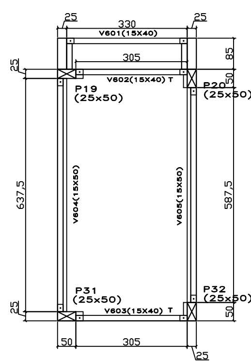
Fôrma Vigas Forro Caixa D'água
