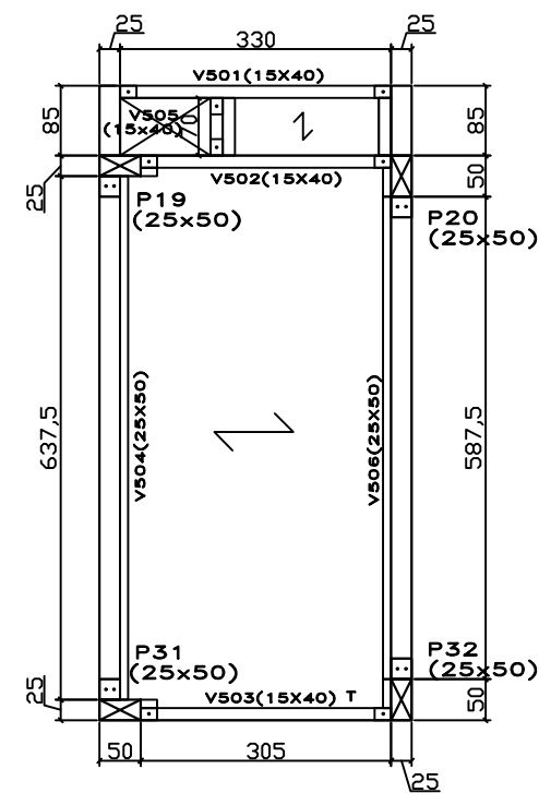
Fôrma Vigas Caixa D'água
